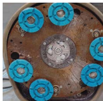
Βήμα 4ο: Γυάλισμα τσιμεντοκονίας με ρητινούχους διαμαντόδισκους.
